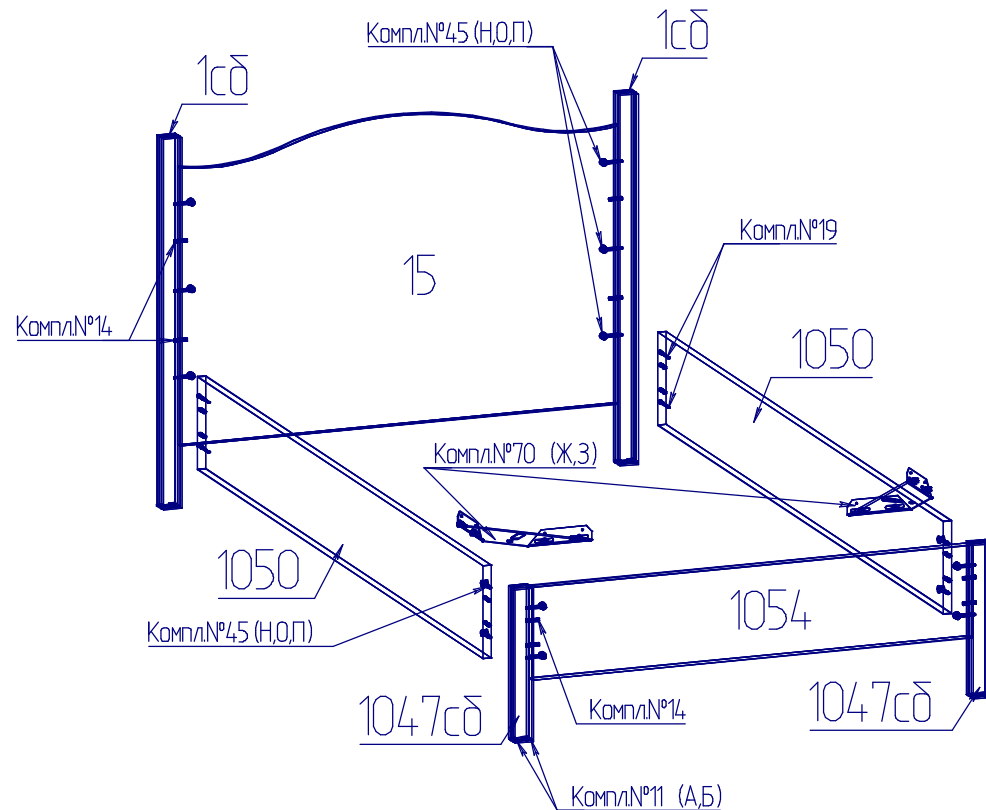
Крепление винта саморезного (комплект №19)
